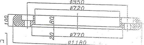
SEC. D-D SC. 1:15
