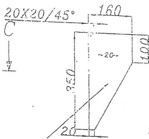
SEC. C-C SC. 1:20
